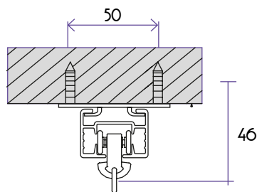
Fissaggio binario a soffitto Ceiling Fix
