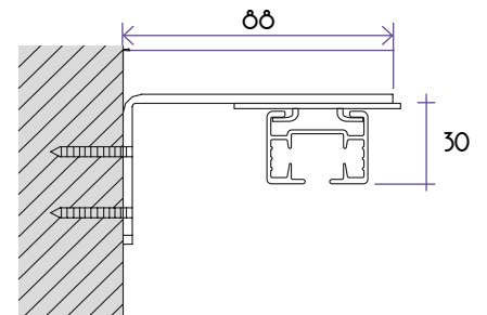
Fissaggio binario a parete Wall Fix
